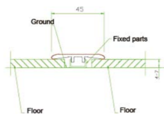
Expansion joint Junta de dilatación
